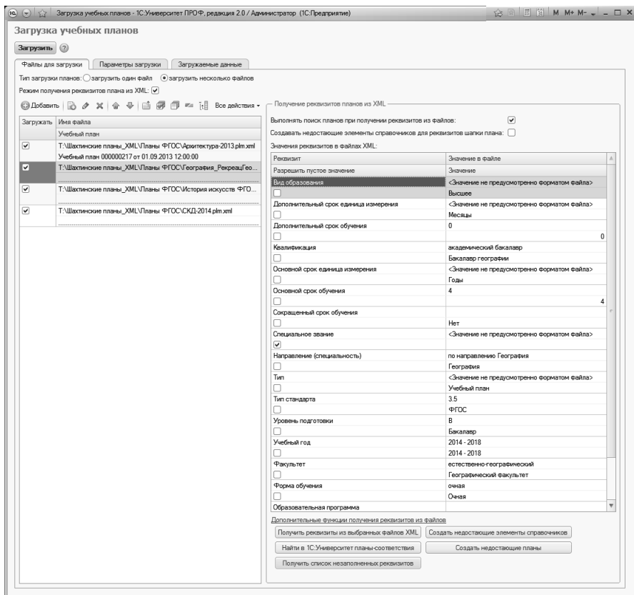
Рис. 38. Форма обработки «Загрузка учебных планов»; вкладка «Файлы для загрузки», массовая загрузка
