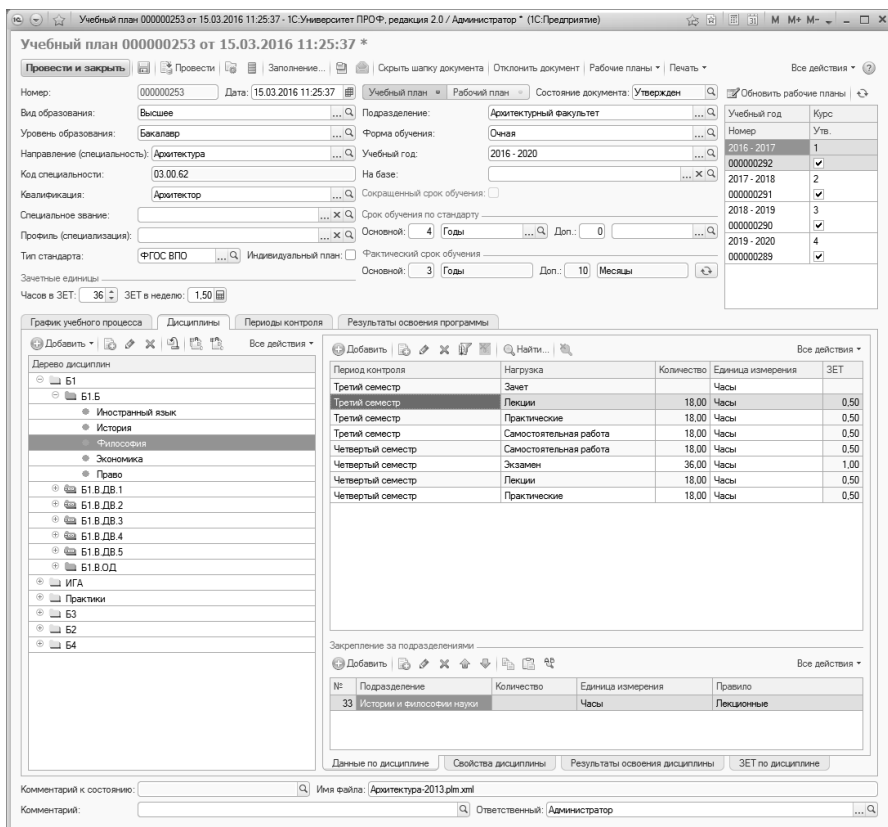
Рис. 25. Форма документа «Учебный план» с активной вкладкой «Дисциплины», данные по дисциплине
